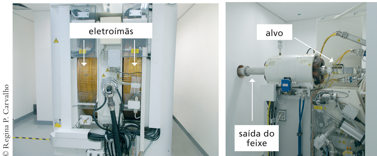
Figura II-3 – Ciclotron (CDTN-CNEN)
